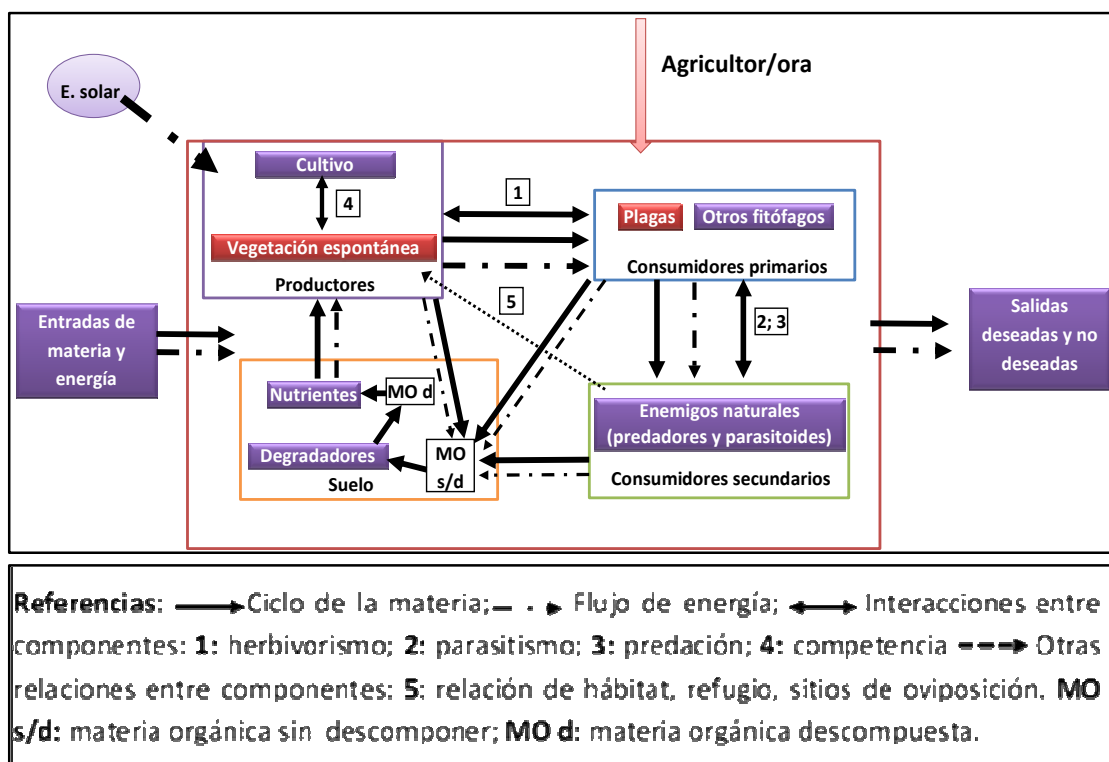
Figura 10.2: Diagrama simplificado de un agroecosistema hipotético: trama trófica, interacciones y relaciones entre componentes, ciclo de la materia, flujo de la energía
