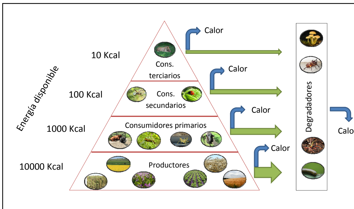
Figura 7.2: Pirámide del flujo de energía. Se supone una pérdida del 10% de la energía utilizable en la transferencia de un nivel trófico al otro
